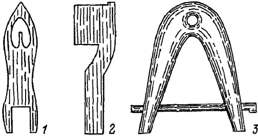
Инструменты для вязания сетей: 1 — игла; 2 — мерка; 3 — вешалка-крючок
