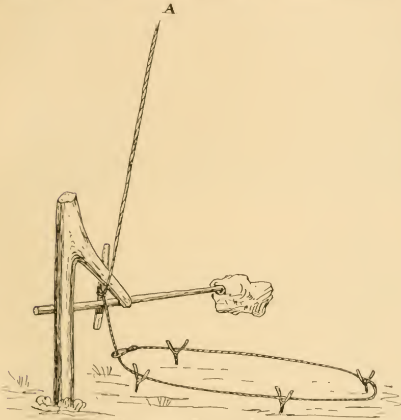
FIG. 16.—Spring snare.
